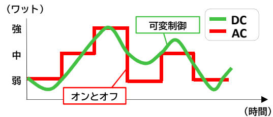
消費電力の動き (イメージ)
