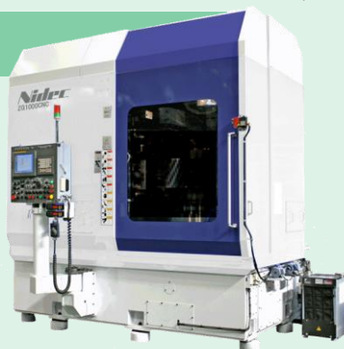
大型歯車研削盤 ZG1000
