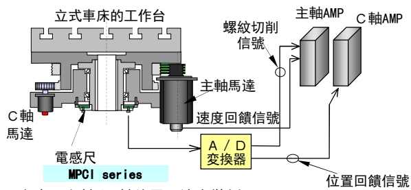
立車 主軸和C軸外置馬達安裝例
