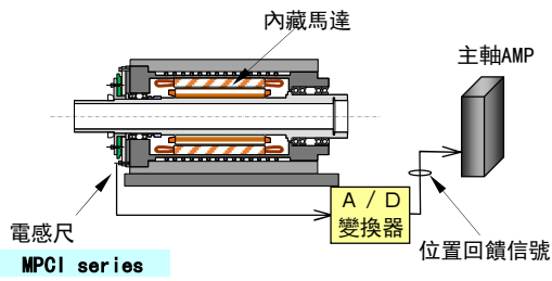
車床 主軸內藏馬達安裝例
