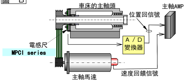
車床 主軸外置馬達安裝例
