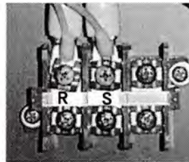
端子台拡大
