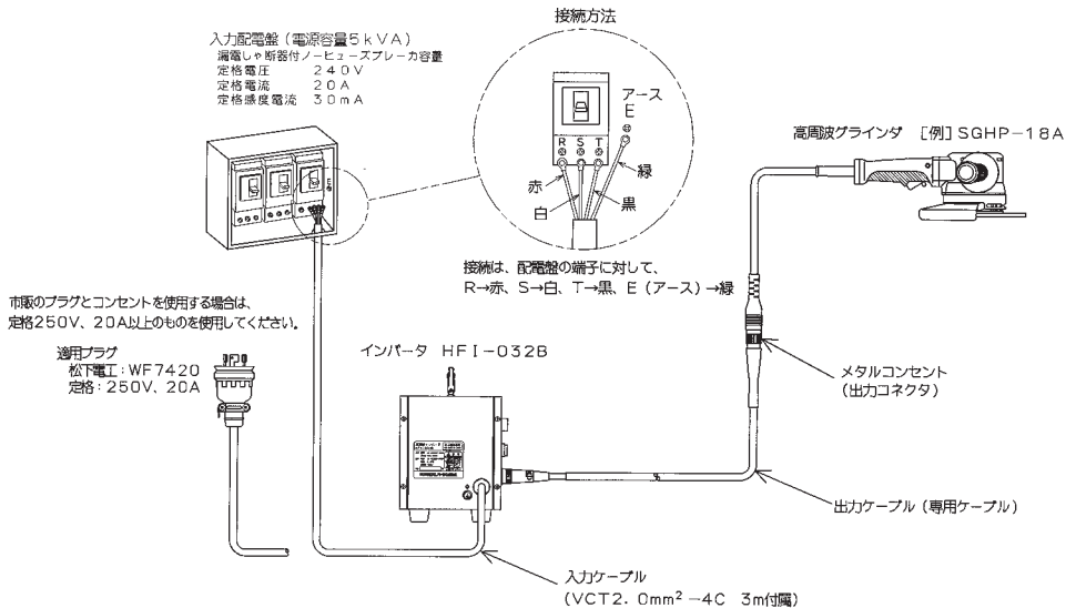
接続図
