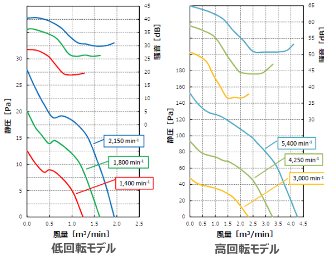
風量-静圧標準特性 (定格電圧)
