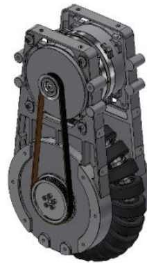
全方位驱动单元 (由本公司与 Honda 共同开发)
