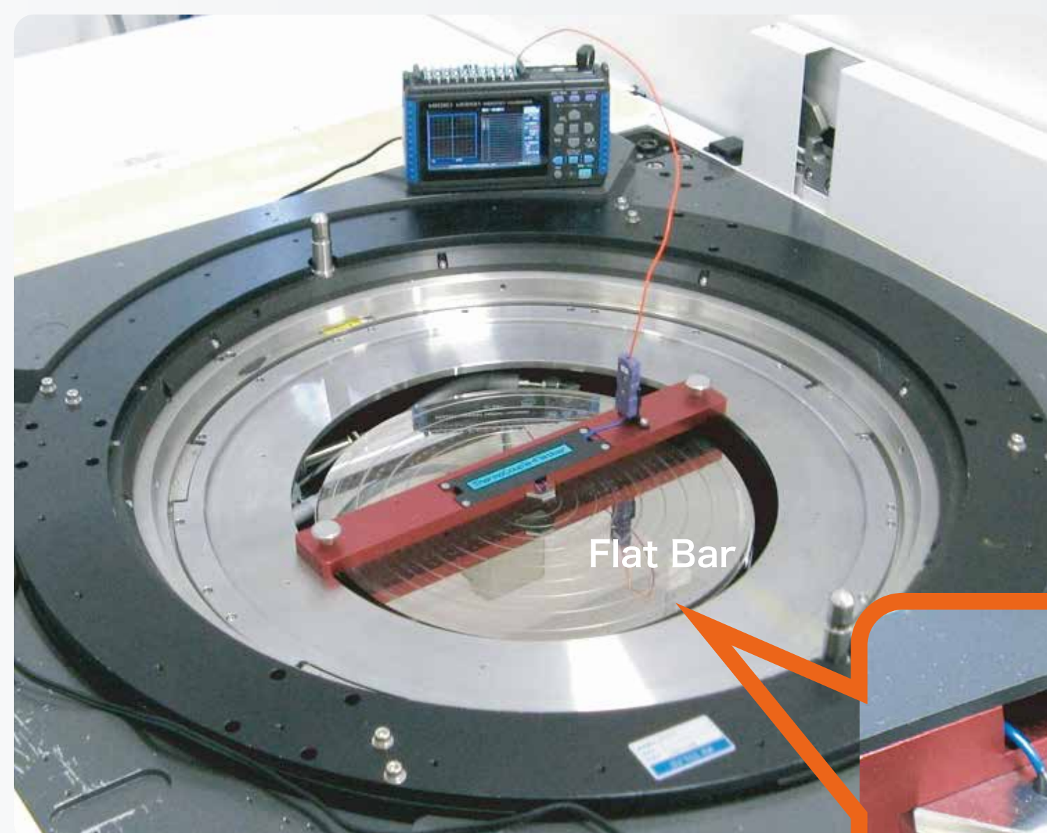
■ Flat Barに組み込んだ場合の使用例 Exaple of use when assembled to the flat bar
