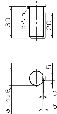
軸端詳細図
