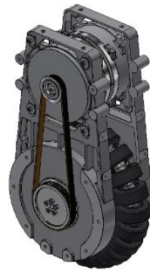
全方位駆動ユニット (当社、Honda 共同開発)
